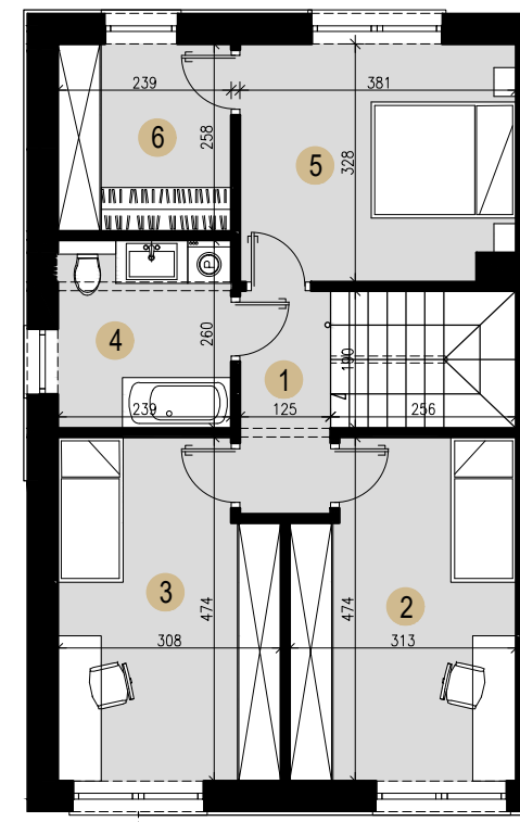
RZUT PIĘTRA
