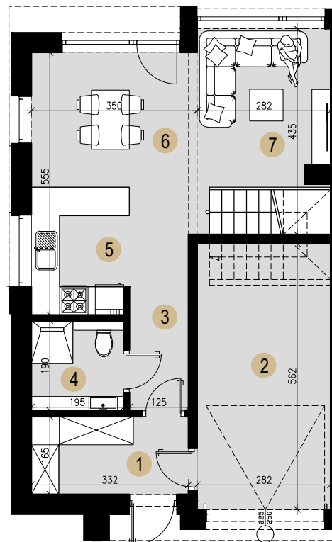
RZUT PARTERU
