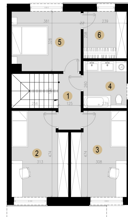
RZUT PIĘTRA
